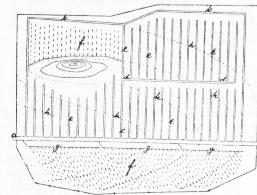
Säännöllinen ojitus suunnitelma. a valtaoja, b niskaoja, c laskuoja, d poikkioja, e sarkaoja (kaikki avo-ojia), f yhdensuuntaisia salaojia (imuojia), g kokoojaoja, h vaakasuorakaarroksia.
